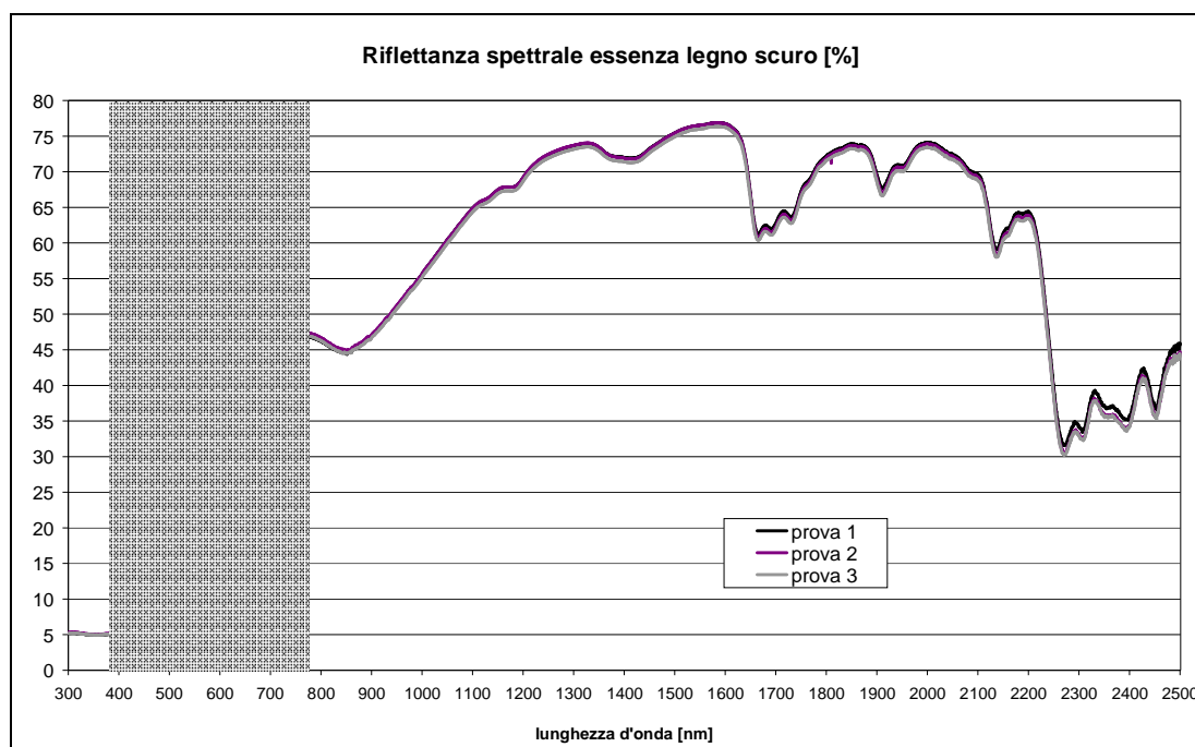
Figura 8 Curve spettrali di tre prove eseguite su una essenza lignea con fondo marrone scuro rifinite con vernice riflettente.
